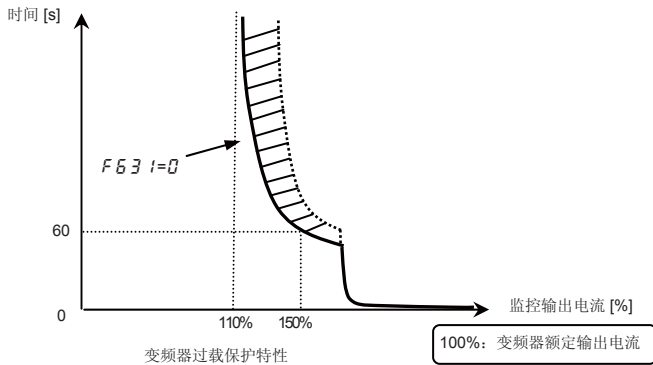
变频器过载保护特性
