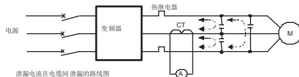
泄漏电流在电缆间泄漏的路线图
