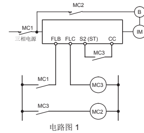
电路图 1
