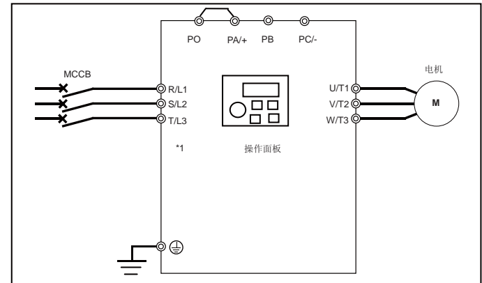
图示 1 操作指令：面板操作 频率指令：设定表盘 1
