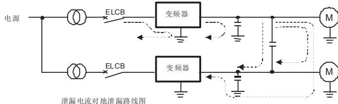
泄漏电流对地泄漏路线图
