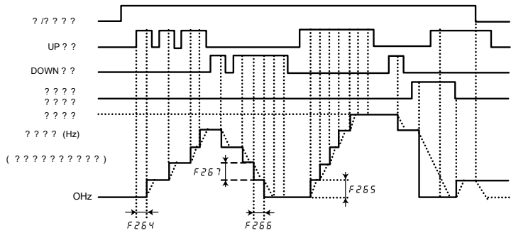
<<序列示例图 2: 通过脉冲信号进行调节>>
