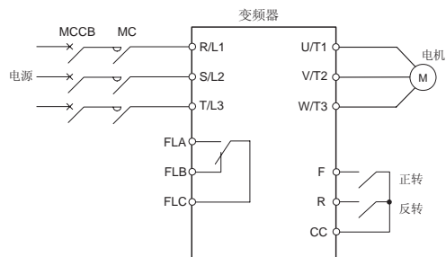
主电路中的磁性接触器接线示例
