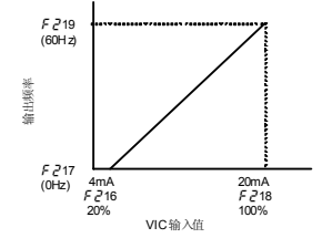
4 - 20 mAdc 电压输入设定示例
