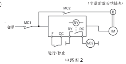
电路图 2
