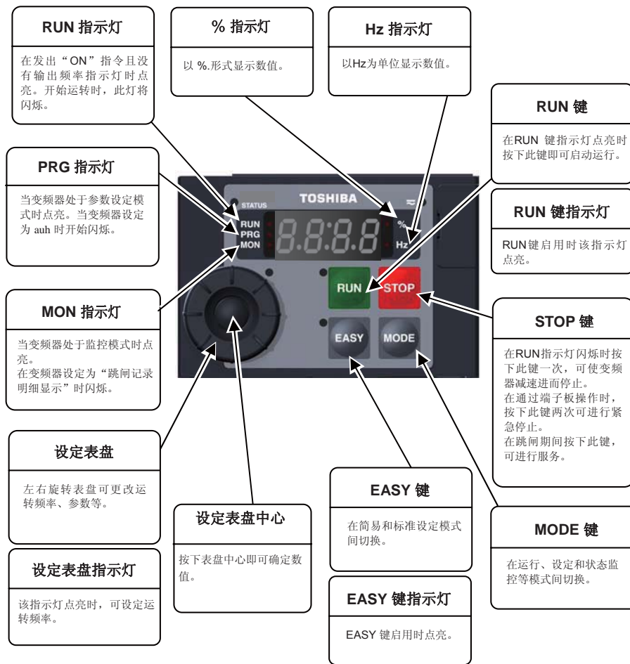
[操作面板]
