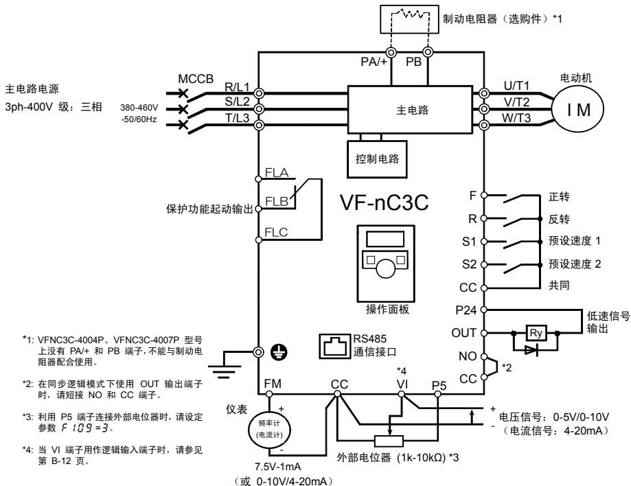
标准连接图-SINK（负极）（通用：CC）
