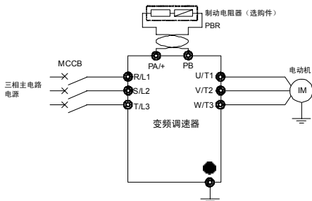
独立选购的电阻器（带热敏保险丝）
