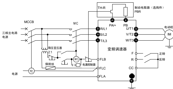
连接热继电器及外部制动电阻器
