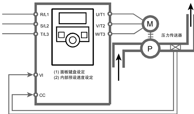
反馈信号 (1) 直流: 4~20mA; (2) 交流: 0~10V; (3) 直流: 0~5V
