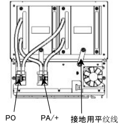
《VFPS1-4500KPC, 4630KPC》
