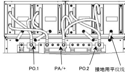
《VFPS1-4500KPC, 4630KPC》
