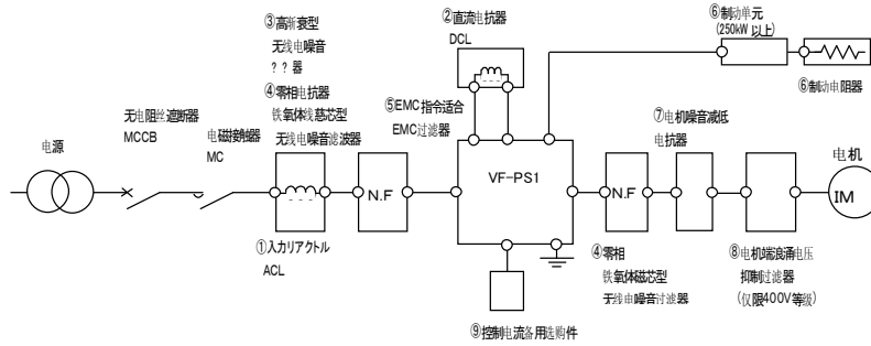
外置式选配件的种类
