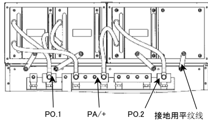
《VFPS1-4400KPC》
