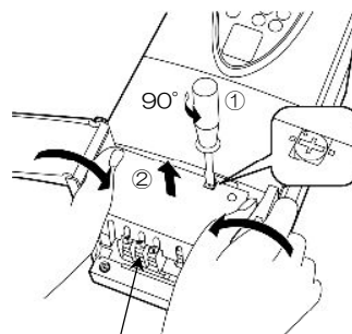
主回路端子台
