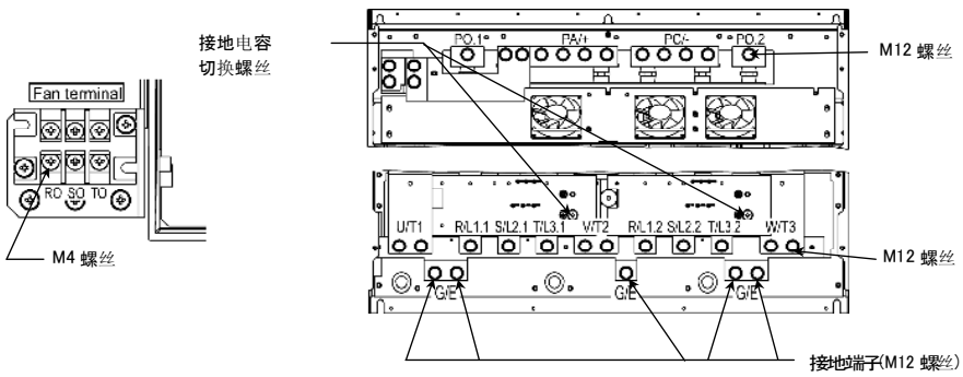
VFPS1-4500KPC
