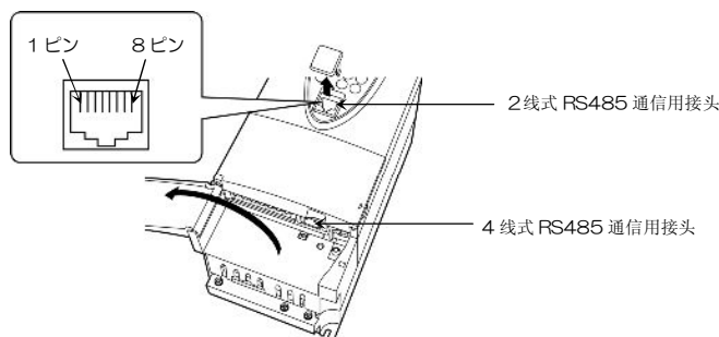
4 线式 RS485
