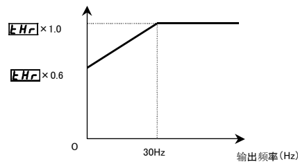
输出电流降低率[%]/[A]
