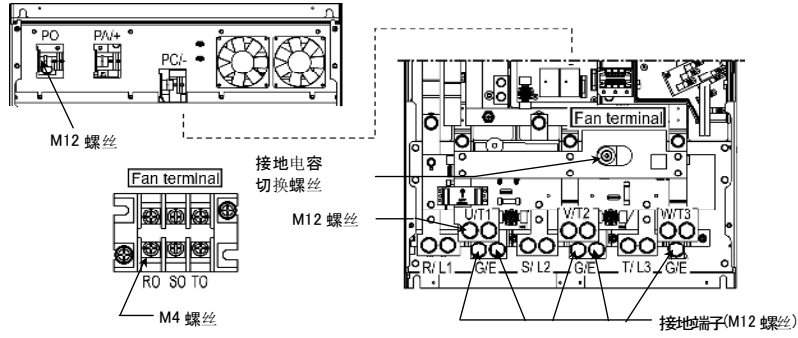
VFPS1-4400KPC
