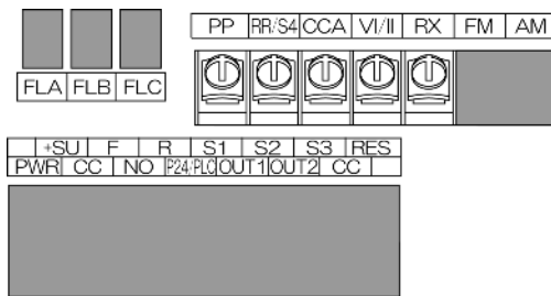
■ 模拟输入端子的功能设定
