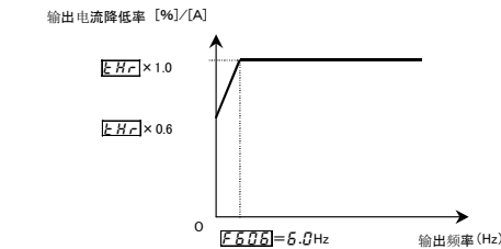
电机过载开始等级的设定
