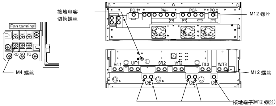
VFPS1-4400KPC
